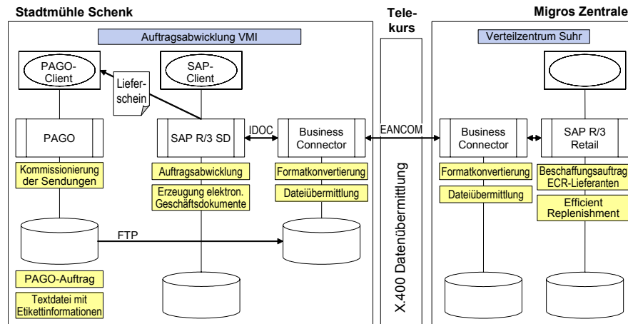
Abb. 14.4: Übersicht über die beteiligten Anwendungssysteme und deren Integration
